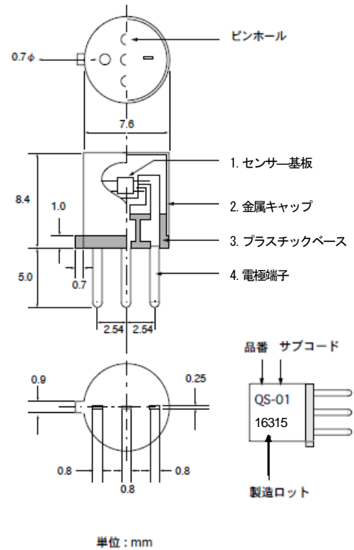
寸法(標準ハウジング)
