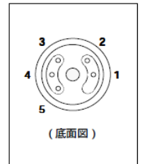
図 1c. 電極端子配置
