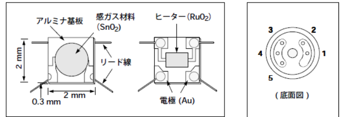
図 1a. 感ガス素子
