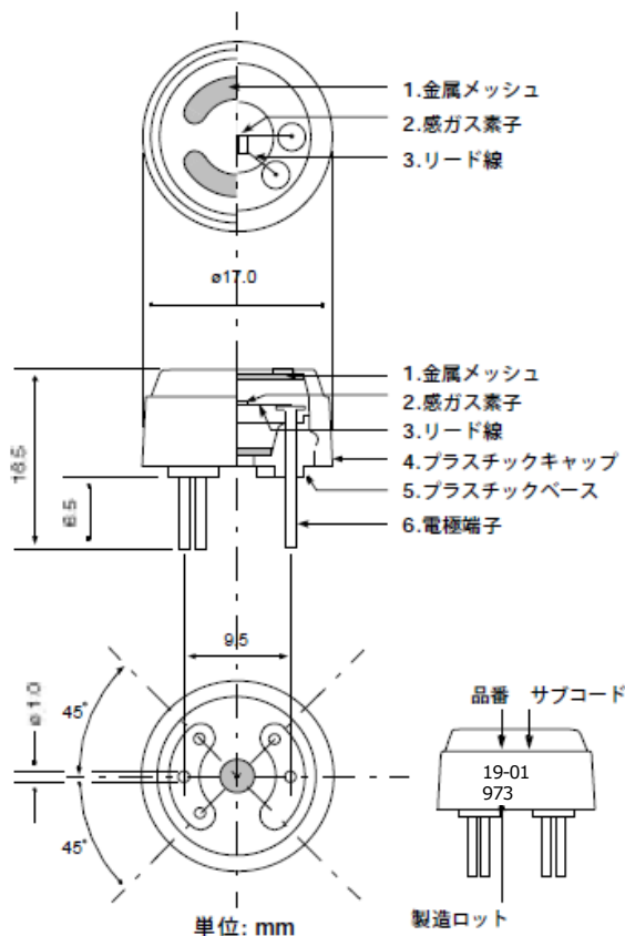
寸法 (標準ハウジング)
