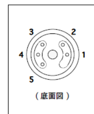
図 1c. 電極端子配置 (底面図)
