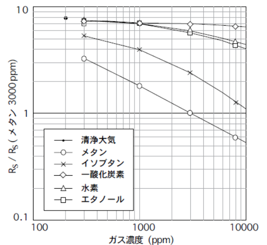
図3. ガス濃度特性
