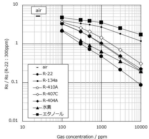
図3. ガス感度特性
