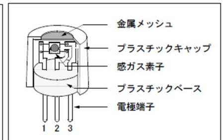
図2. センサー構造
