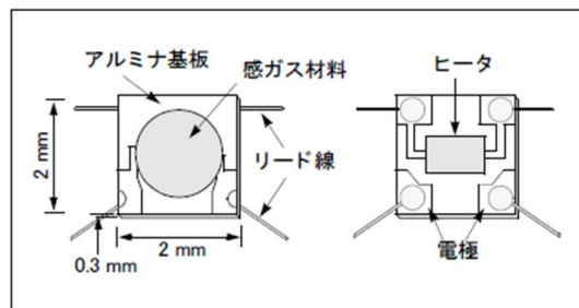
図1. 感ガス素子
