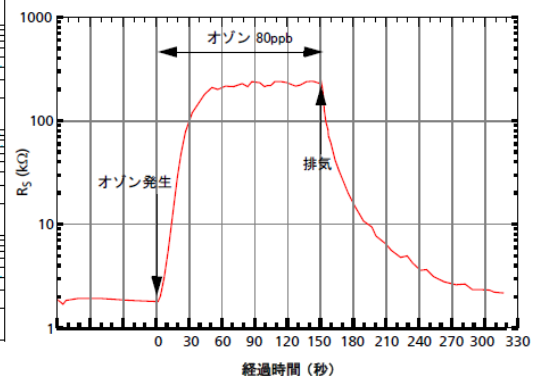
図4. ガス応答性
