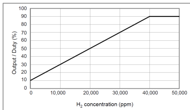
図 1. モジュール出力特性
