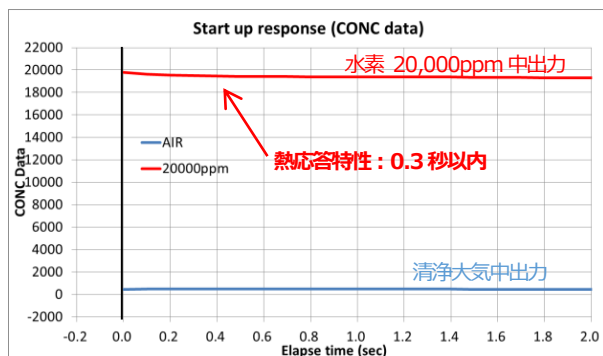
図 2. ガス応答性
